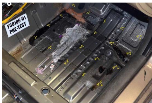
FIGURA 55. Pré-Teste - Chapa de Assoalho no Lado do Passageiro
