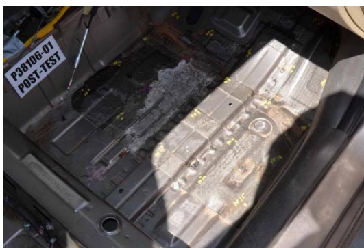
FIGURA 56. Pós-Teste - Chapa de Assoalho no Lado do Passageiro
