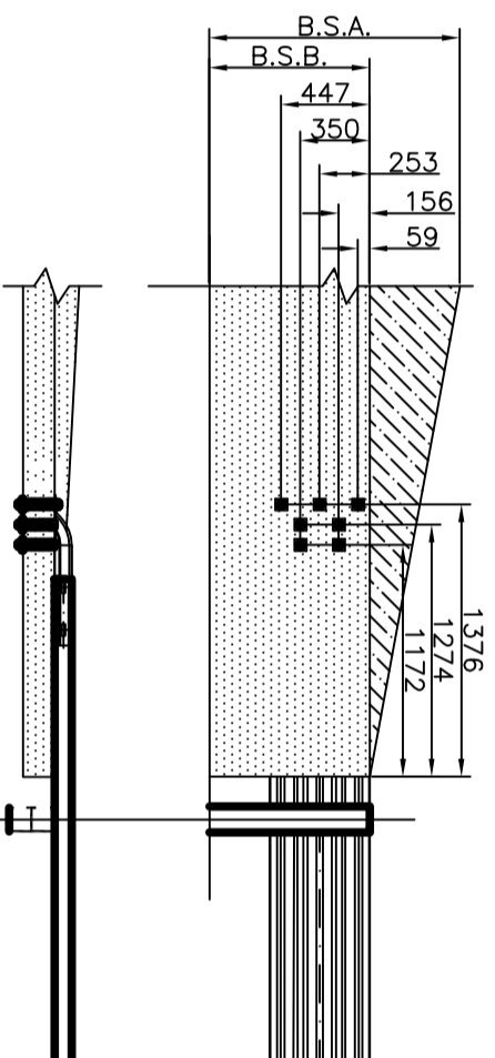
DETALHE DA CONEXÃO COM O ELEMENTO RIGIDO
